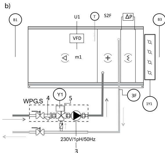
Рис.1. Схема подключения узла регулирования полностью собранного WPG (a) и простой конфигурации WPG.S (b) к агрегату для вентиляции и кондиционирования воздуха
