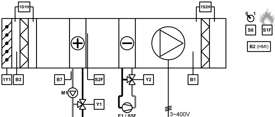
Схема управления NS 5
